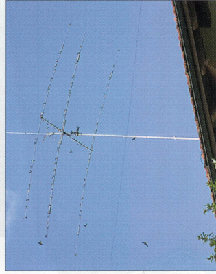
Eine drehbare Richtantenne; ein sog. Beam, die Querelemente sind ca. 8 m lang; hier offensichtlich gar für Vögel ein beliebiger Aufenthaltsort
