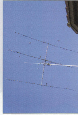
Antenne directive orientable appelée «beam», un beau perchoir pour les oiseaux; les éléments transversaux mesurent env. 8 m
